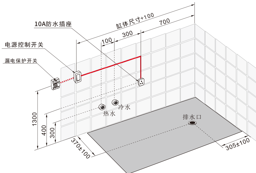
水电安装尺寸图
